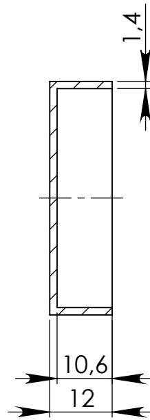
PRZEKRÓJ A-A
