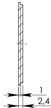
PRZEKRÓJ B-B
